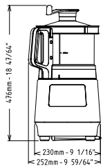
Zij aanzicht
